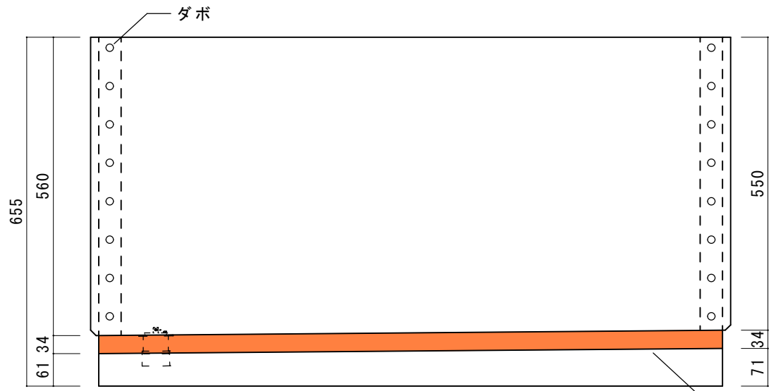
底板木口銅板貼
